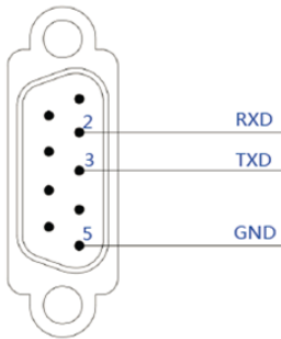
COM1/2/3-RS232 接口定义
